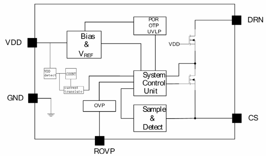
功能框图
